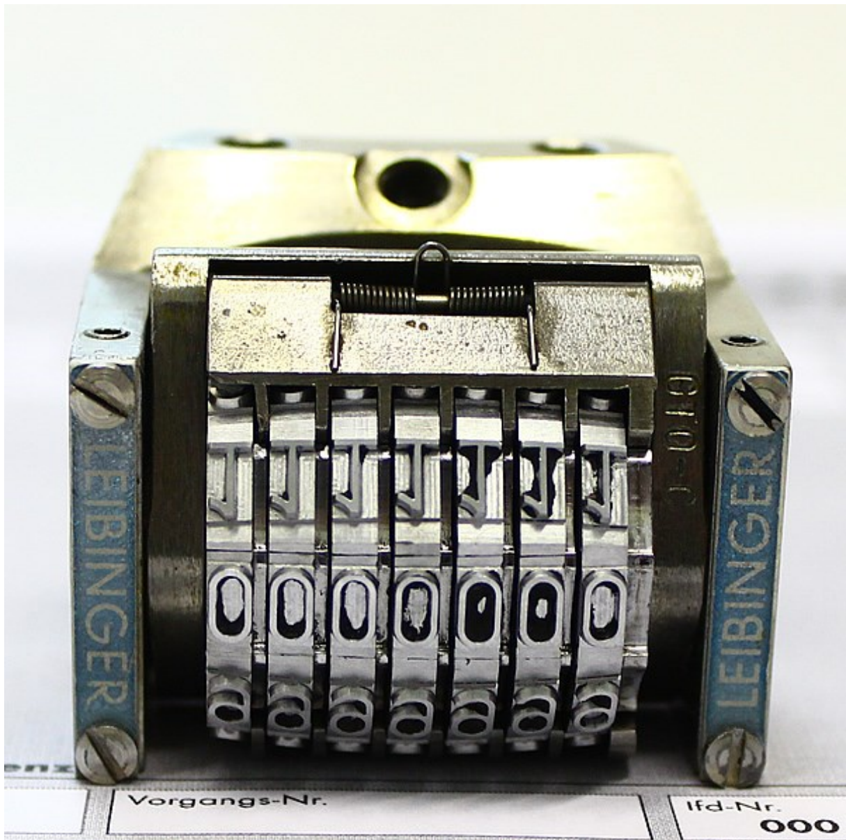
Abbildung: Nummerierwerk
